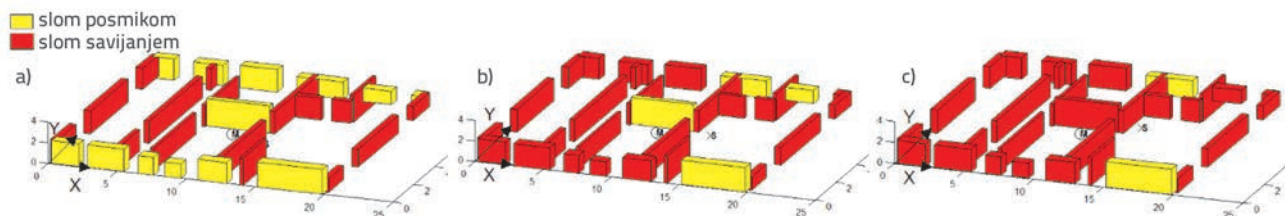
Slika 12. Načini sloma kod graničnog stanja nosivosti u smjeru x, određeni pomoću programa SREMB: a) prije injektiranja; b) nakon injektiranja s LC1; c) nakon injektiranja s C1
