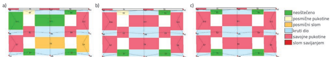
Slika 13. Načini sloma kod graničnog stanja nosivosti u smjeru y (zapadni fasadni zid), određeni pomoću programa 3MURI: a) prije injektiranja; b) nakon injektiranja pomoću smjese LC1; c) nakon injektiranja pomoću smjese C1
