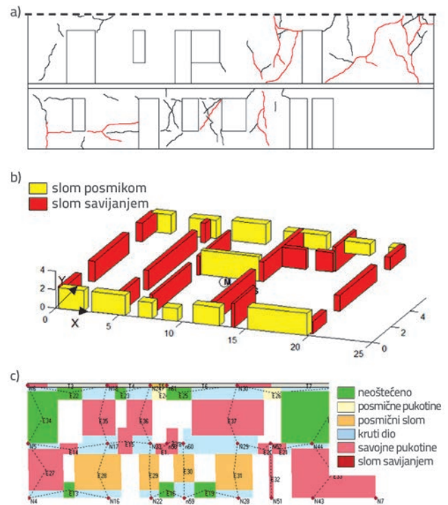
Slika 11. Oblik pukotina registriran na južnoj fasadi: a) usporedba sa slomom u graničnom stanju opterećenja prema modelu SREMB; b) prema modelu 3MURI; c) nearmirano stanje
