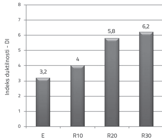
Slika 6. Indeks duktilnosti
