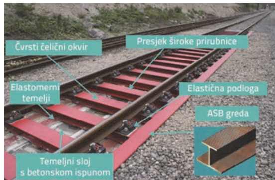
Slika 8. Dvoslojni metalni sustav kolosijeka
