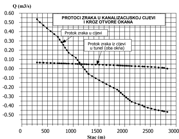
Slika 4. Protoci zraka u kanalizijskoj cijevi i kroz otvore okana
