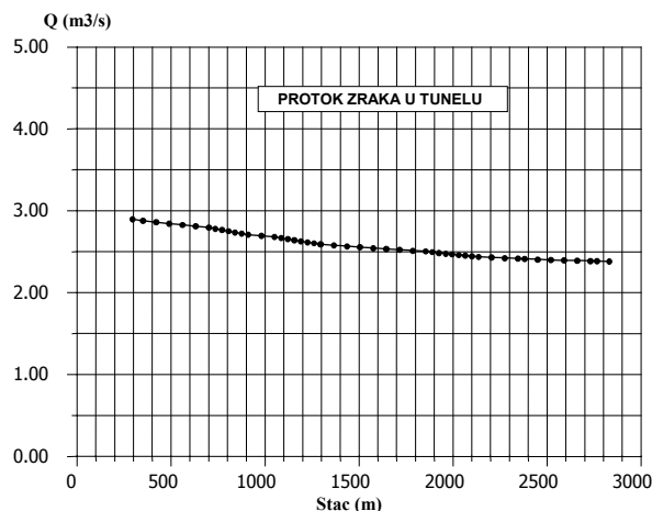
Slika 10. Protok zraka u tunelu
