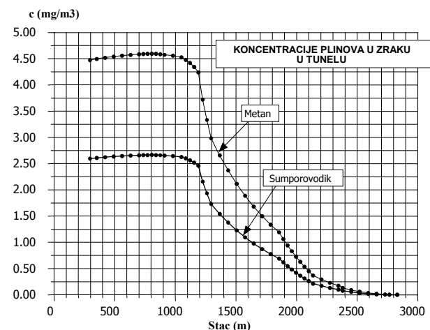
Slika 13. Koncentracije plinova u zraku u tunelu.
