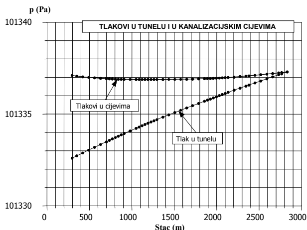
Slika 11. Tlakovi u tunelu i u kanalizacionjskim cijevima
